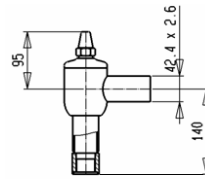
EA32/G1"-I
